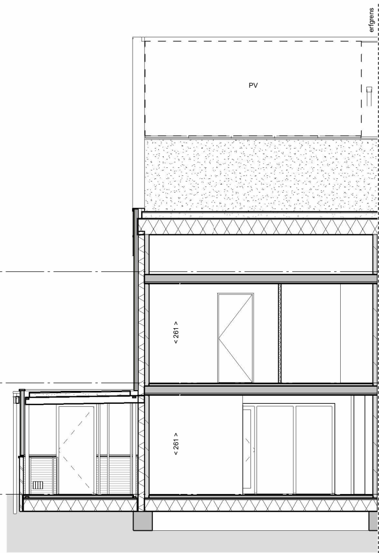
langsdoorsnede
