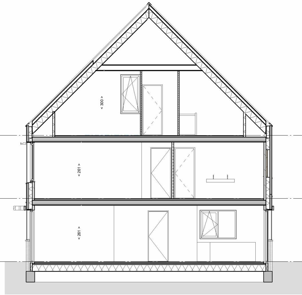
dwarsdoorsnede
