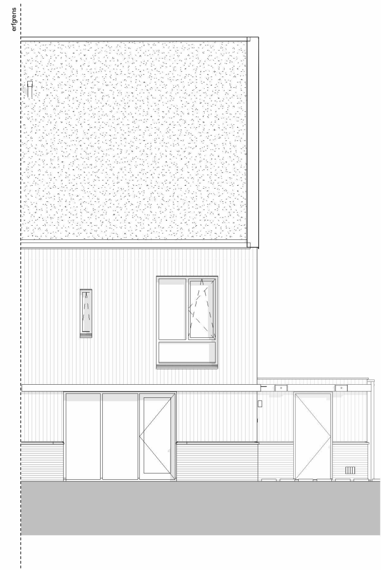
voorgevel (noord)
