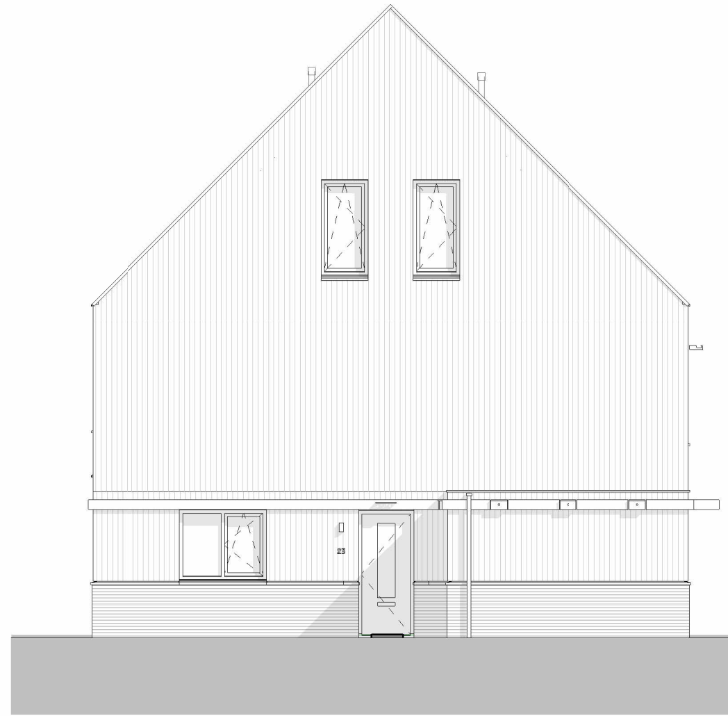
zijgevel (west)
